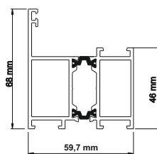
Profil progów ENERGY 60
