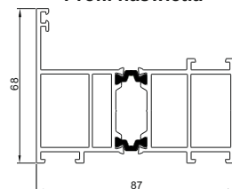
Profil progów ENERGY 90
