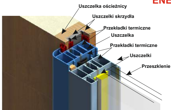
SKRZYDŁO KMT PLUS 75 passive PROFIL OŚCIEŻNICY ENERGY 90 + PROFIL NAŚWIETLA
