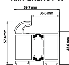
Profil ościeżnicy KMT ENERGY 60
