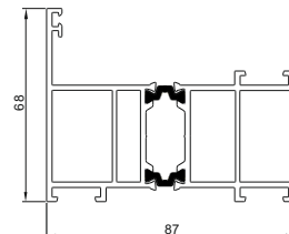
Profil progu ENERGY 90
