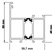
Profil progu ENERGY 60
